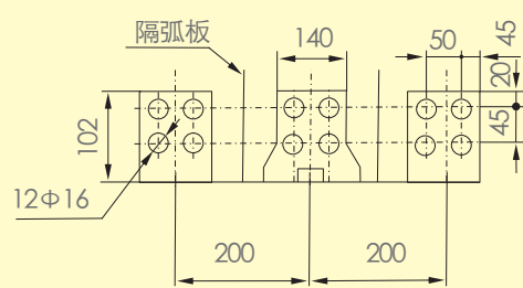
小4000型3级抽屉式水平接线
