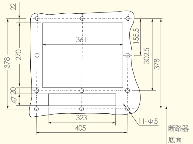
柜门开孔和安装孔距
