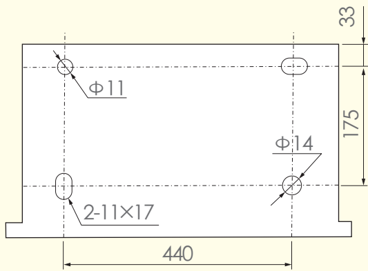
安装尺寸图
