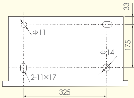
安装尺寸图
