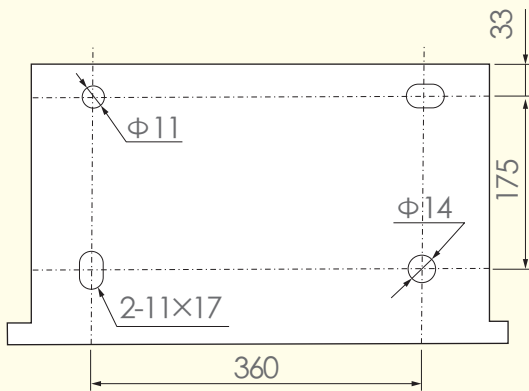
安装尺寸图
