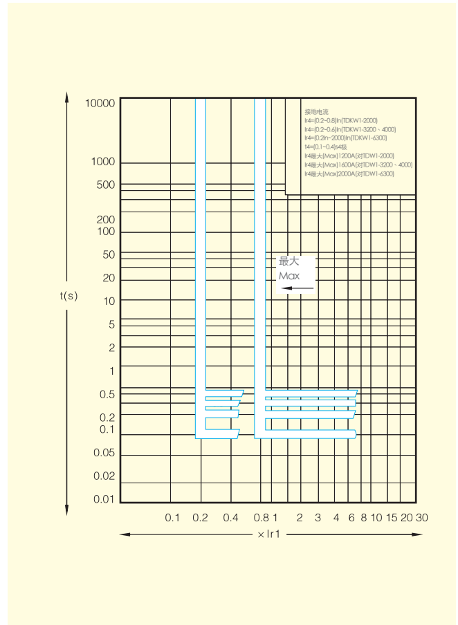
HiPro 6.0 / HiPro 7.0 智能控制器接地故障保护时间 电流特性曲线
