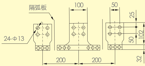
小4000型3级固定式水平接线
