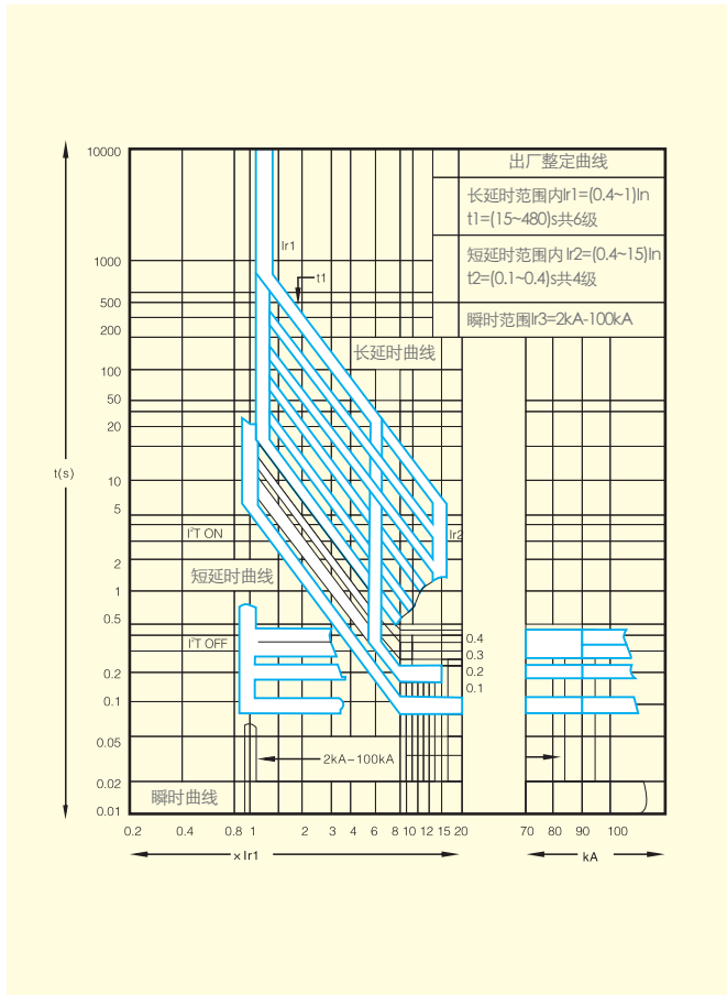
HiPro 6.0 / HiPro 7.0 智能控制器时间 电流特性曲线
