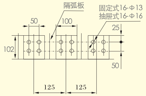
3200型3P水平接线
