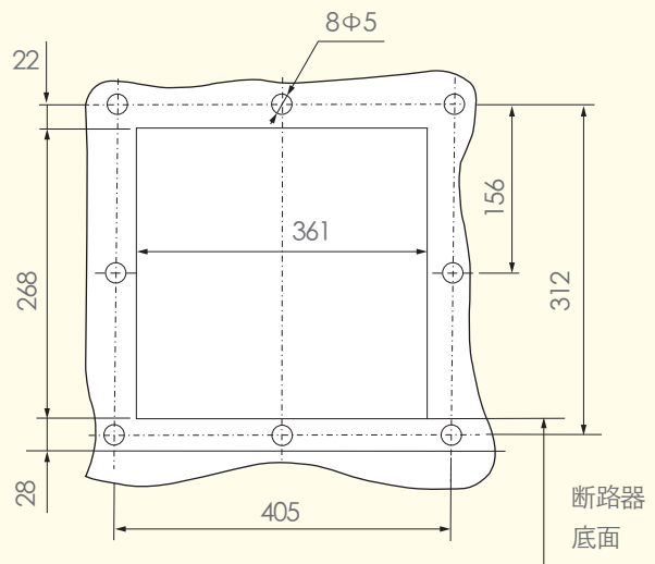
柜门开孔和安装孔距
