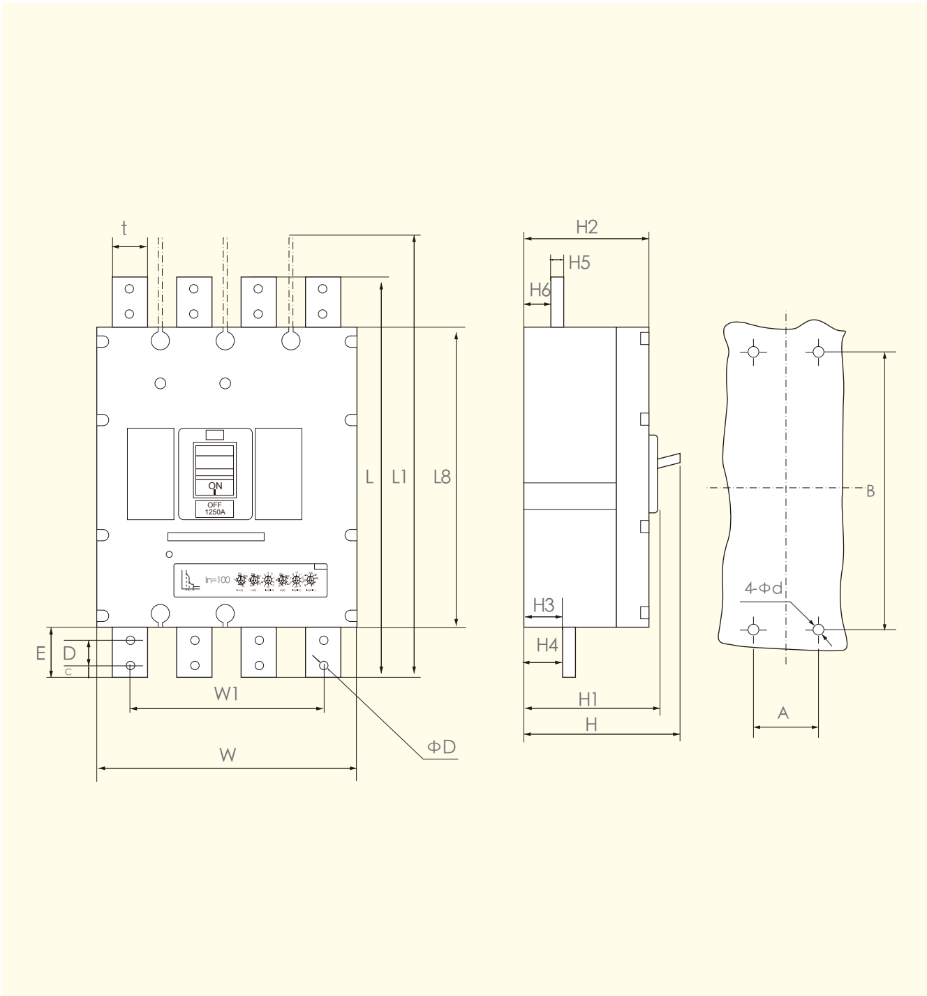
1250/1600外形尺寸及安装尺寸
