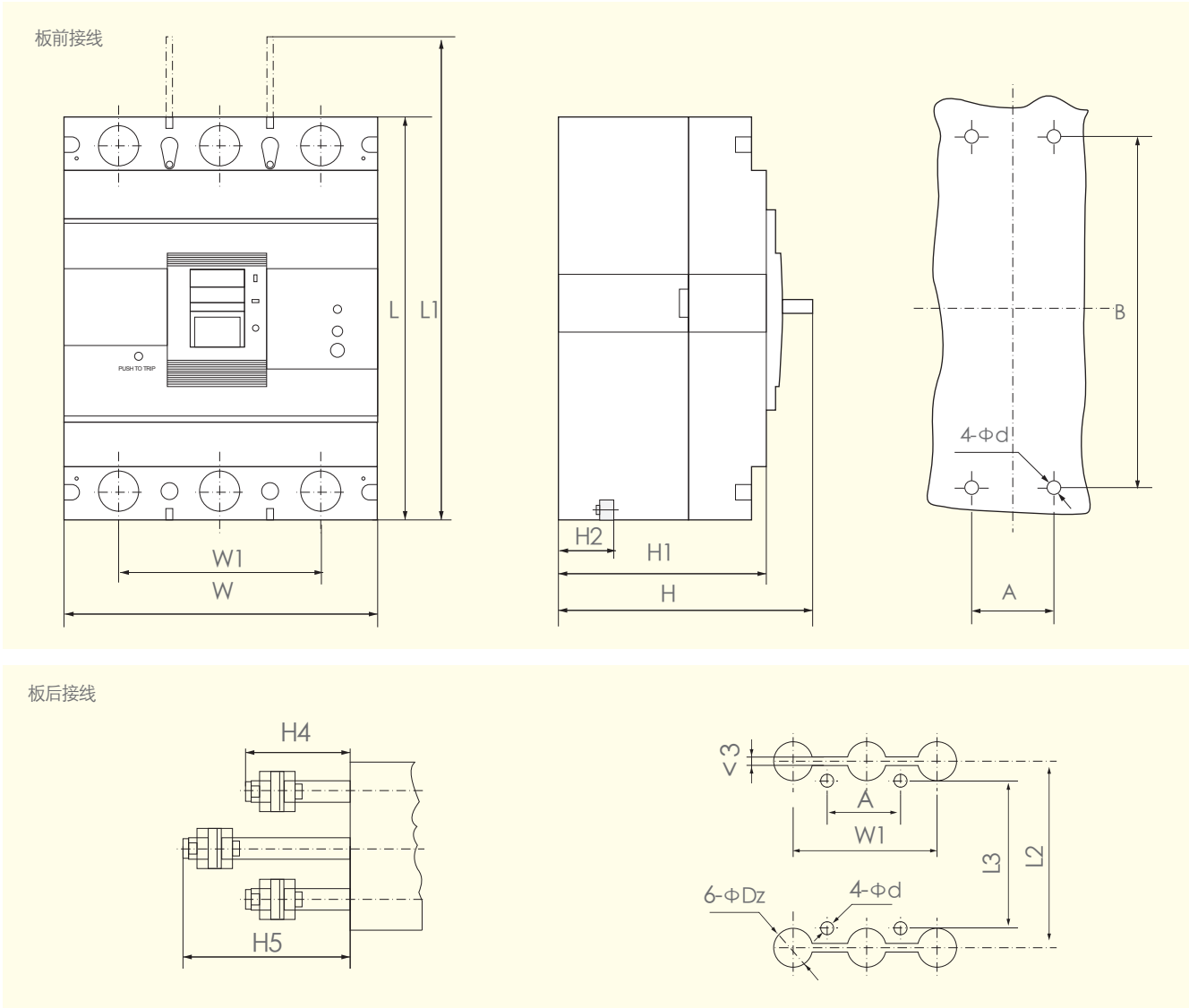
塑壳漏电空气断路器 外形尺寸及安装尺寸
